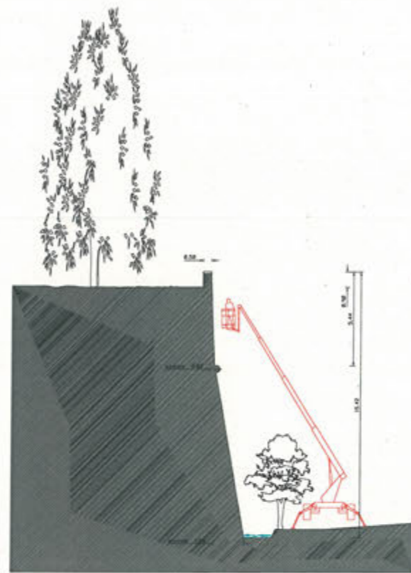
SEZIONE 2
