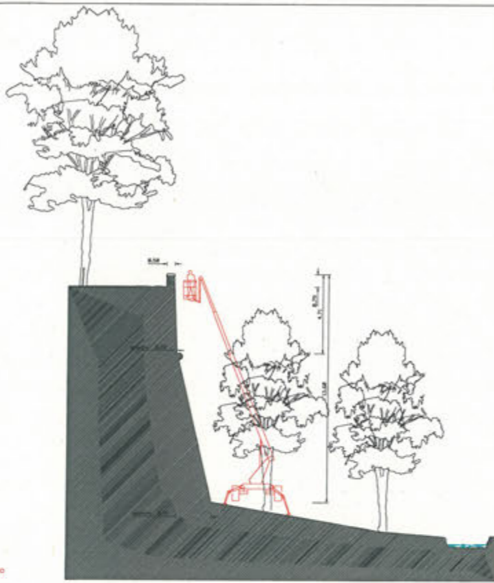
SEZIONE 1
