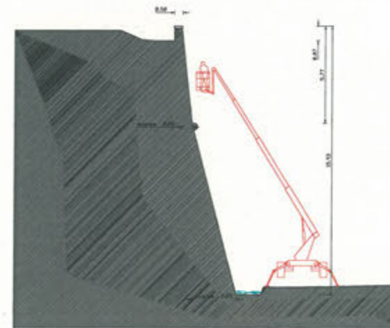
SEZIONE 3
